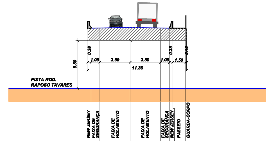
SEÇÃO TIPO 4 - PASSAGEM SUPERIOR
