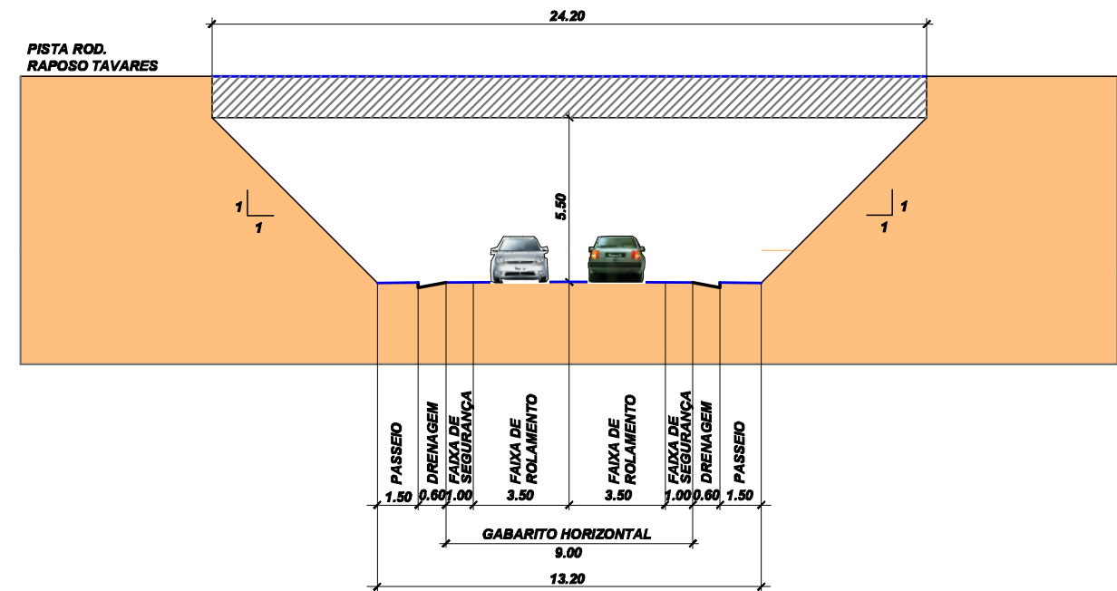
SEÇÃO LONGITUDINAL DE PASSAGEM INFERIOR
